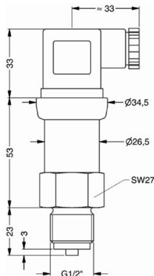
G1/2" EN 837
